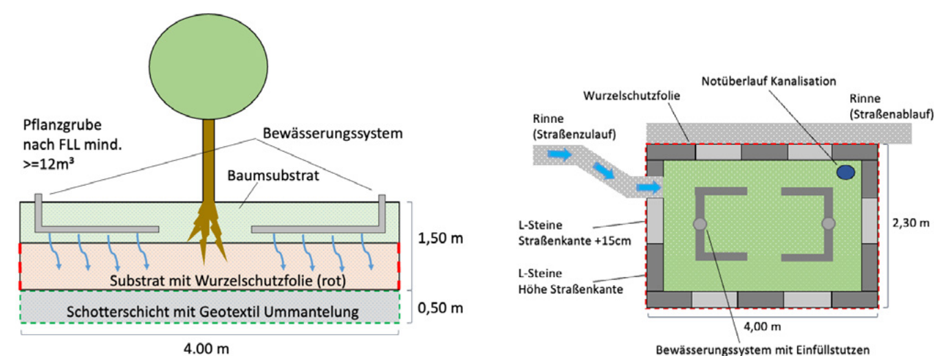
Abb. 83: Schematischer Profilschnitt durch eine Pflanzgrube und als Aufsicht (Klimaanpassungsmanagement Landkreis Darmstadt-Dieburg 2026)
