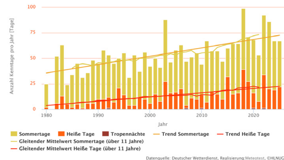
Abb. 28: Anzahl der Ereignistage (Sommertage, Heiße Tage sowie Tropennächte) aufgezeichnet an der Klimastation Schaafheim-Schlierbach im Betrachtungszeitraum 1980-2025 (HLNUG 2025a)
