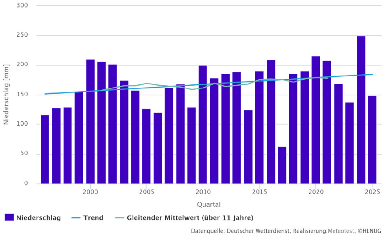
Abb. 36: Zeitliche Entwicklung der Niederschläge im Winter (Dezember-Februar) an der Klimastation Darmstadt im Betrachtungszeitraum 1996-2025 (HLNUG 2025a)
