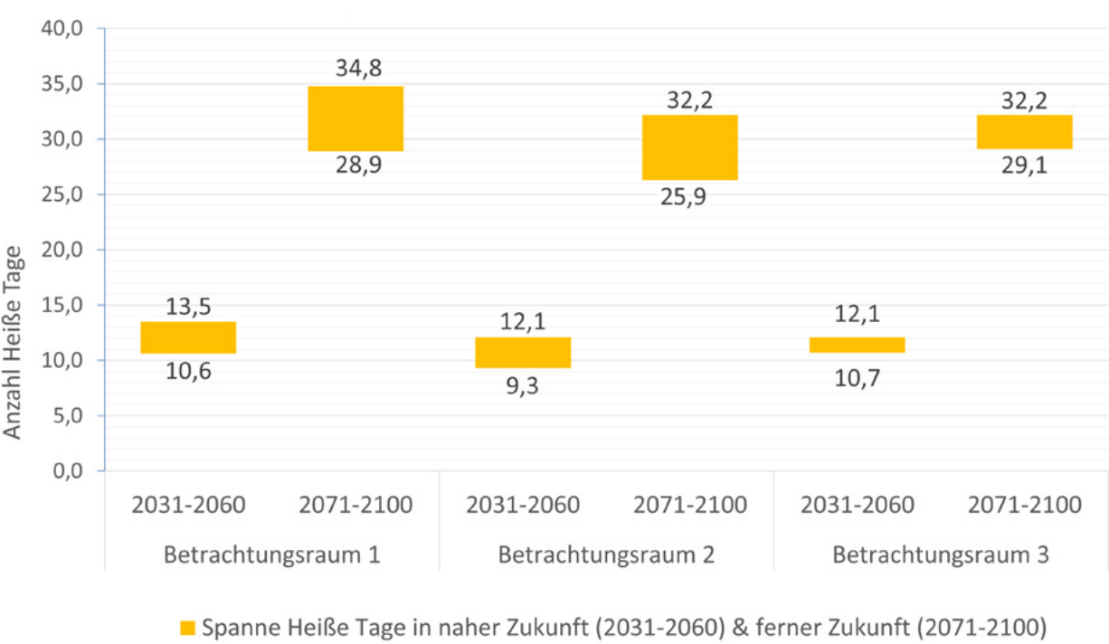
Abb. 47: Projizierte Änderungen der mittleren Anzahl an Heißen Tagen nach dem RCP 8.5-Szenario für die Kommunen im Landkreis Darmstadt-Dieburg – nahe Zukunft und ferne Zukunft (INFRASTRUKTUR & UMWELT 2026, basierend auf: HLNUG 2025d)
